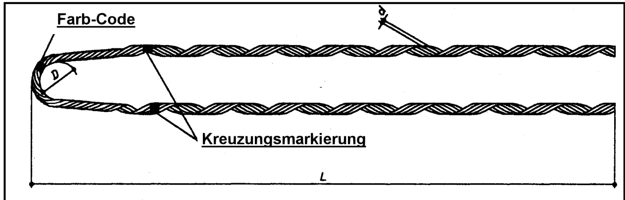
Abspannschnecke
