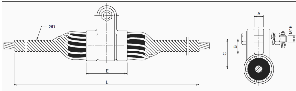
Spiraltragklemme
