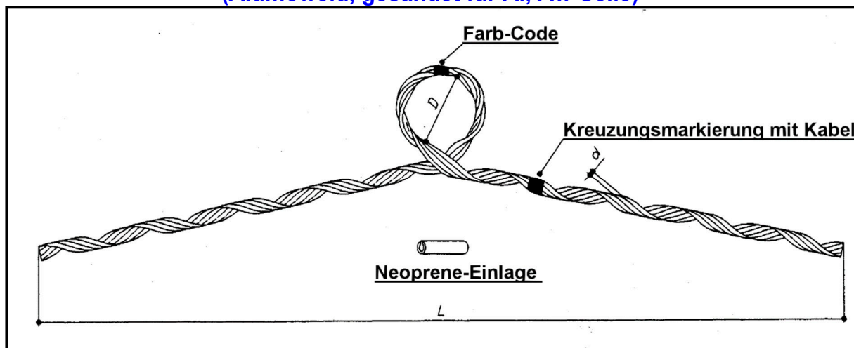
Seitenbundspirale
