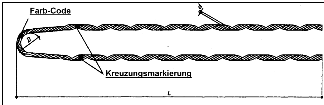
Abspannspirale
